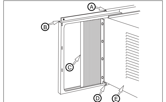
(A) Barra superior (D) Barra inferior (B) Marco del panel de relleno (E) Gabinete (C) Borde de fijación
