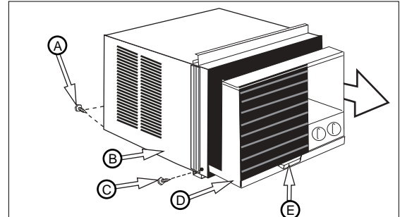
(A) Tornillos de embarque (D) Chasis (B) Gabinete (E) Manija de la bandeja inferior (C) Tornillos antirrobo
