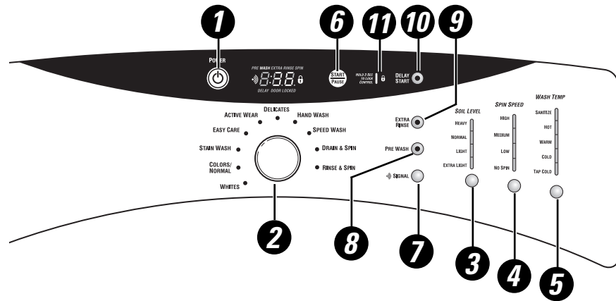
Modelo WBVH6240
