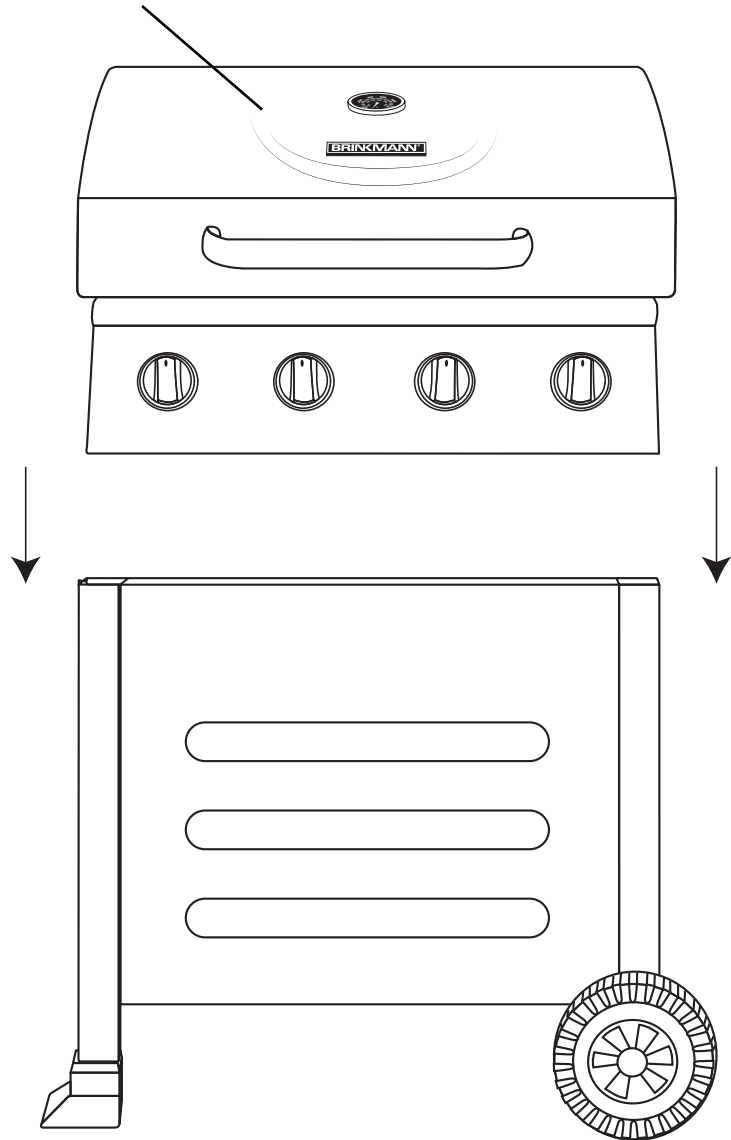
Montaje del Cuerpo de la Parrilla
