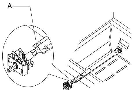
A. Raccordement brûleur/gicleur
