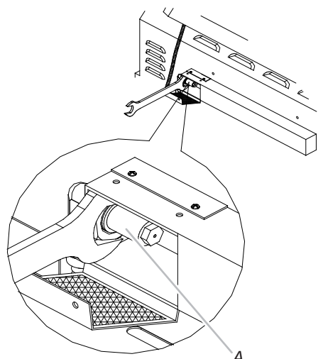
A. Tuerca del orificio
