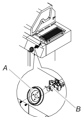
A. Cerclage B. Tige de réglage
