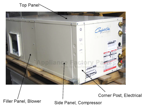
HRH Sheetmetal Parts
