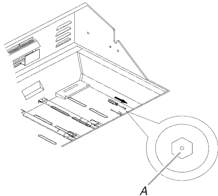
A. Orificio
