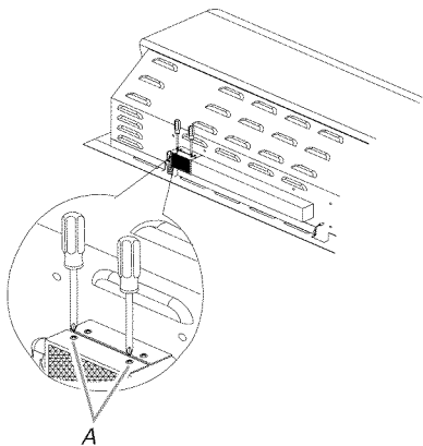
A. 2 tornillos
