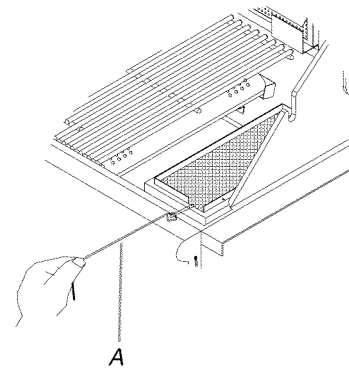
A. Porte-allumette
