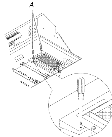
A. 2 screws
