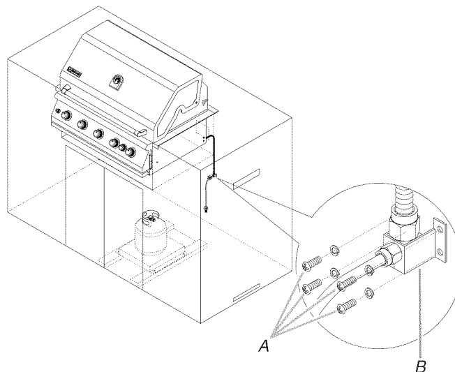
A. 4 vis B. Support de montage à bride laiton 90° en 2 parties
