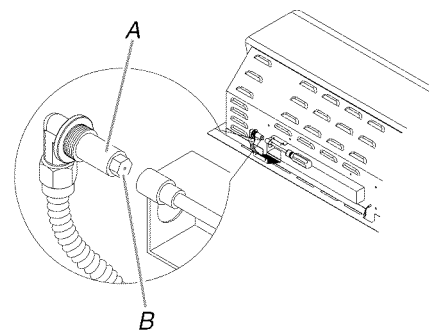
A. Support de gicleur B. Gicleur
