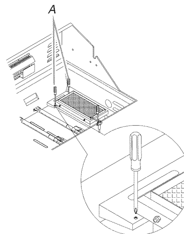
A. 2 tornillos
