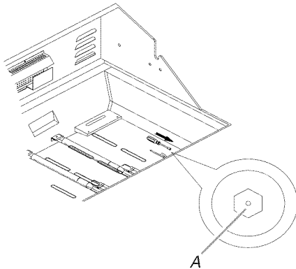
A. Orifice
